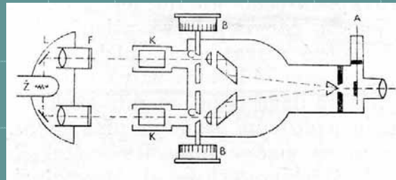
Pulfrichův fotometr a jeho schéma
